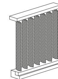
D11 - Frangisole verticale. Angoli prestabiliti e variabili. Collegabile frontalmente e lateralmente allamuratura ed alle sottostrutture in acciaio. D11 - Vertical sunblades. Preset and variable angles. Can be connection frontally and laterally to the wall and to the steel substructure.
